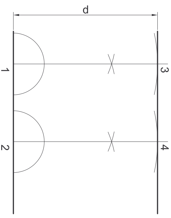
PARALLELA AD UNA RETTA ALLA DISTANZA d
