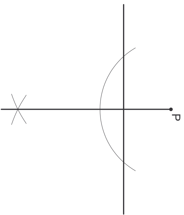
Perpendicolare ad una retta per un punto non app. ad essa
