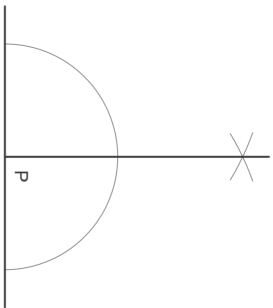
Perpendicolare ad una retta per un suo punto
